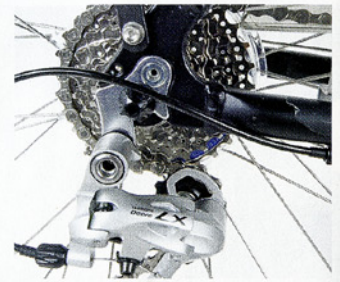
Austauschbares Ausfallende: Im Schadensfall bleibt der Rahmen verschont
